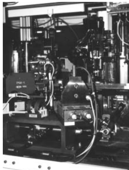
自社製電気マイクロメータを使用した測定部 Measuring station with our original “Electronic Gages”.
