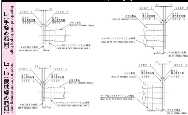
●管とゲージとの関係図 Related positions of pipe and gauges
