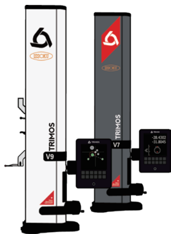
高性能縦型測長機 V9/V7 シリーズ
