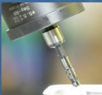
空気マイクロメータで 内径・外径を測定
