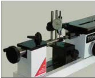
テストインジケータの検査 (THV-100 / THV-150)
