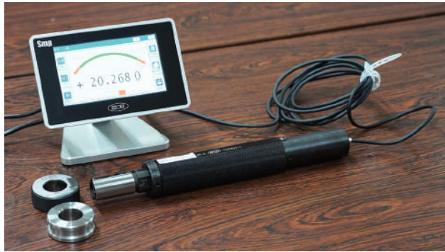
内径測定 (ボアゲージ使用)
