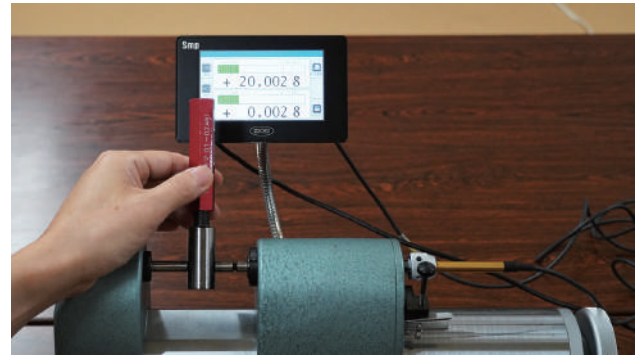
外径測定 (比較測長機使用)
