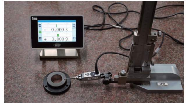
平行度測定 (てこ式プローブ使用)
