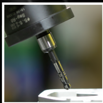
空気マイクロメータで 内径を測定
