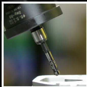
空気マイクロメータで 内径測定
