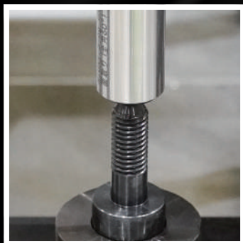
ねじリングゲージで おねじの通り検査
